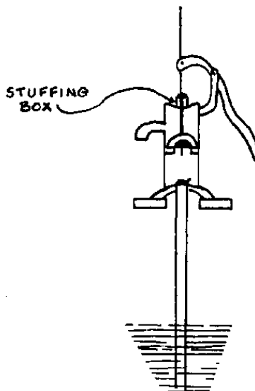
FIG. VII-5. NON-EXTRACTABLE CYLINDER & FIG. VII-6. EXTRACTABLE CYLINDER
