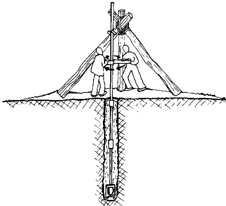
FIG. 12-1. HAND AUGERING
