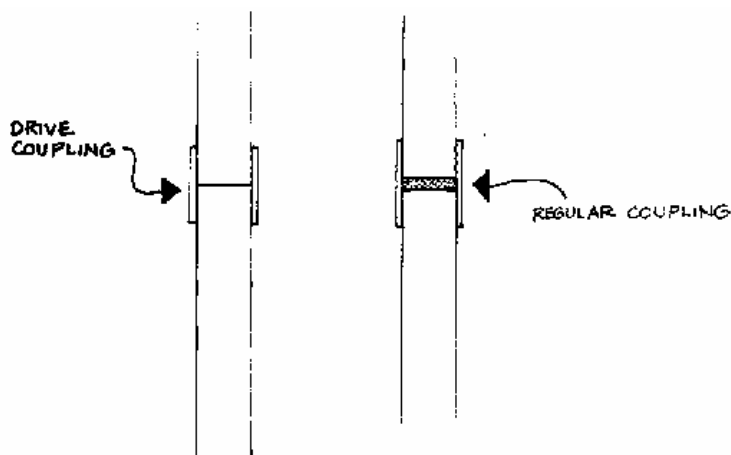
FIG. 14-3. PIPE COUPLINGS
