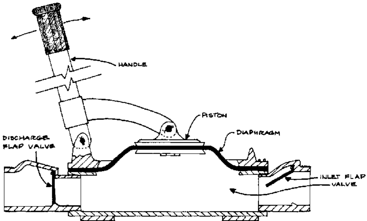
FIG. VII-9. DIAPHRAGM PUMP
