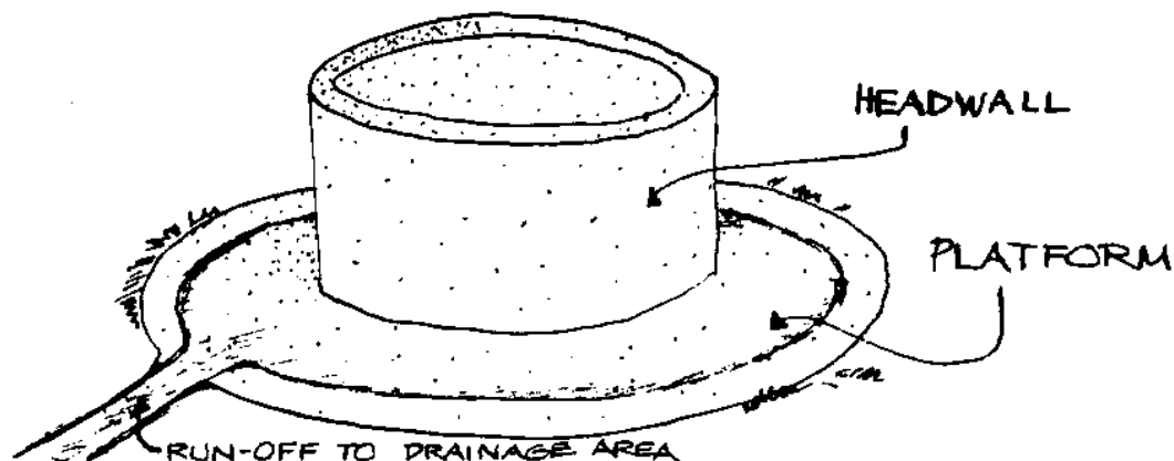
FIG. 3-7. TOP SECTION
